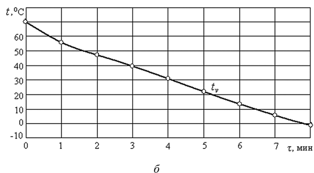
Рис. 3. Кривые изменения температуры (а) на поверхности ( t_{\text{пов}} ) и в центре ( t_{\text{ц}} ) моркови слоем толщиной \delta = 0,01 м и средневolumной температуры ( t_{\text{у}} ) (б) при охлаждении газообразным азотом с температурой t_{\text{ср}} = -40 °C и скоростью его циркуляции \omega_{\text{ср}} = 5 м/с
