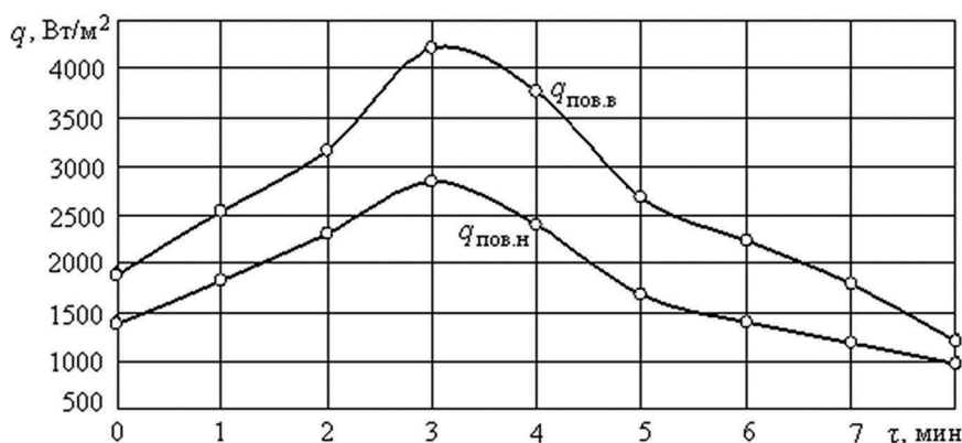
Рис. 4. Кривые изменения плотности теплового потока ( q ) на верхней ( q_{\text{пов.в}} ) и нижней ( q_{\text{пов.н}} ) поверхностях слоя моркови толщиной \delta = 0,01 м при охлаждении газообразным азотом с температурой t_{\text{ср}} = -40 °С и скоростью его циркуляции \omega_{\text{ср}} = 5 м/с
