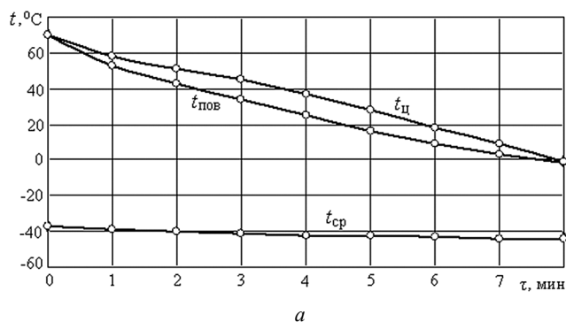
Рис. 3. Кривые изменения температуры (а) на поверхности ( t_{\text{пов}} ) и в центре ( t_{\text{ц}} ) моркови слоем толщиной \delta = 0,01 м и средневolumной температуры ( t_{\text{у}} ) (б) при охлаждении газообразным азотом с температурой t_{\text{ср}} = -40 °C и скоростью его циркуляции \omega_{\text{ср}} = 5 м/с
