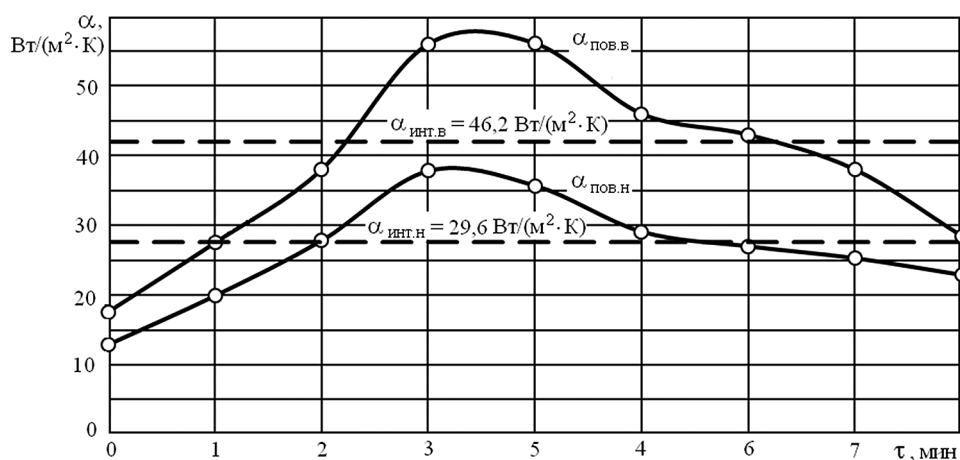
Рис. 5. Кривые изменения коэффициента теплоотдачи \alpha = f(\tau) для верхней ( \alpha_{пов.в} ) и нижней ( \alpha_{пов.н} ) поверхностей слоя моркови толщиной \delta = 0,01 м при охлаждении газообразным азотом с температурой t_{ср} = -40 °С и скоростью его циркуляции \omega_{ср} = 5 м/с: \alpha_{инт.в} и \alpha_{инт.н} — средние интегральные значения параметра, Вт/(м 2 ·К)
